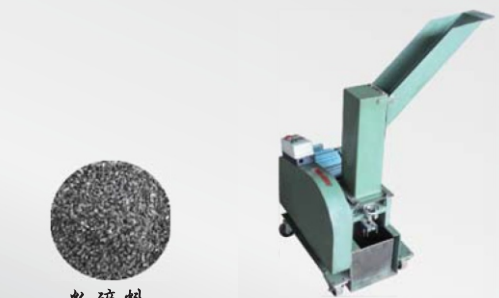
粉碎机 grinder
