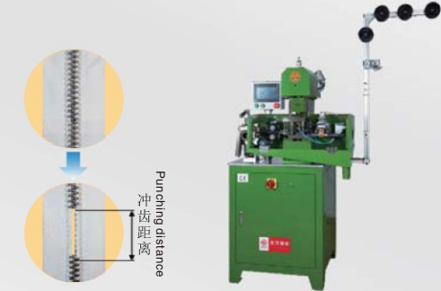
全自动金属冲齿机(单选齿) automatic metal zipper gapping machine
