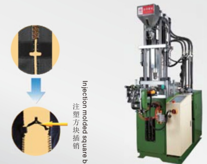
全自动开口注塑机 fully automatic open end pin & box machine
