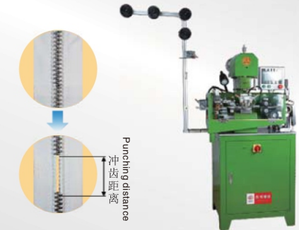
全自动金属冲齿机(双选齿) automatic metal zipper gapping machine
